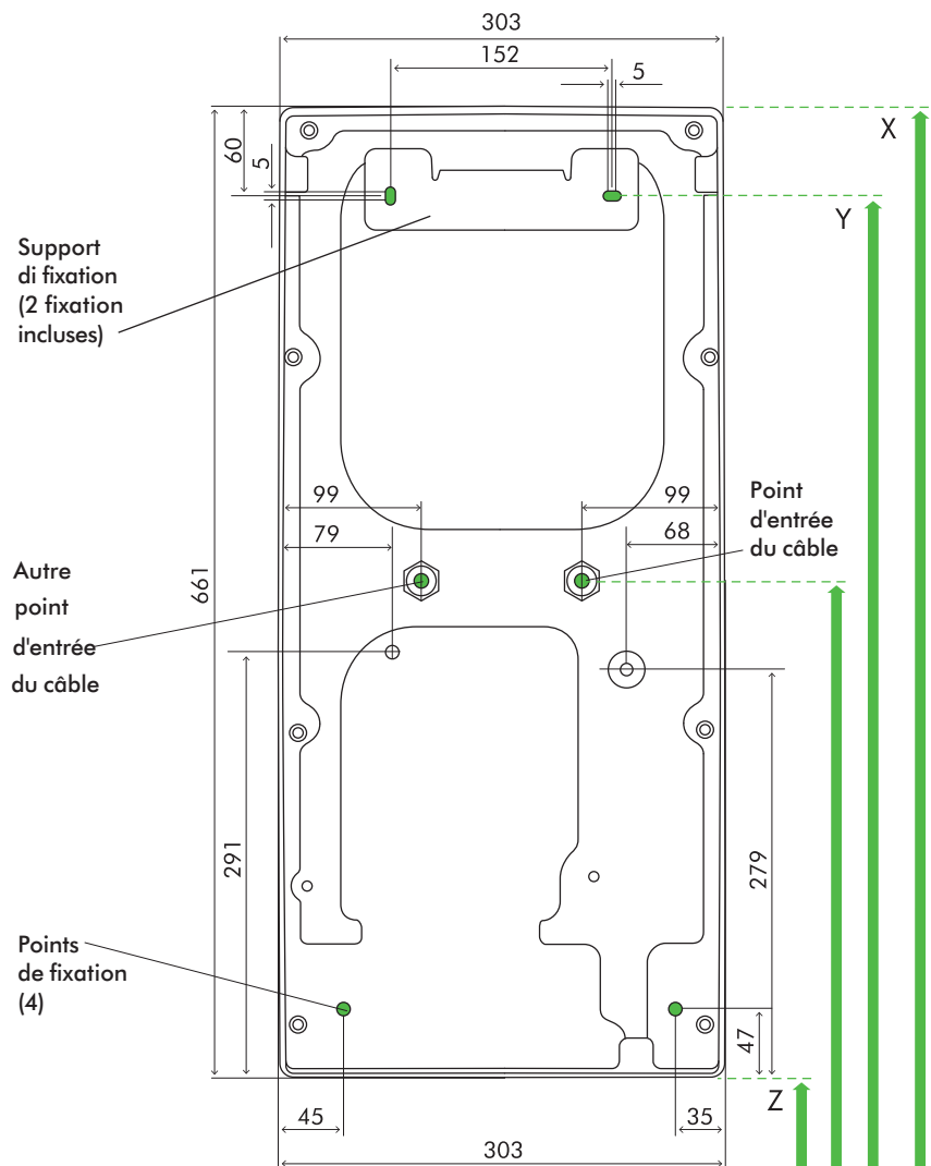
ÉLÉVATION ARRIÈRE
